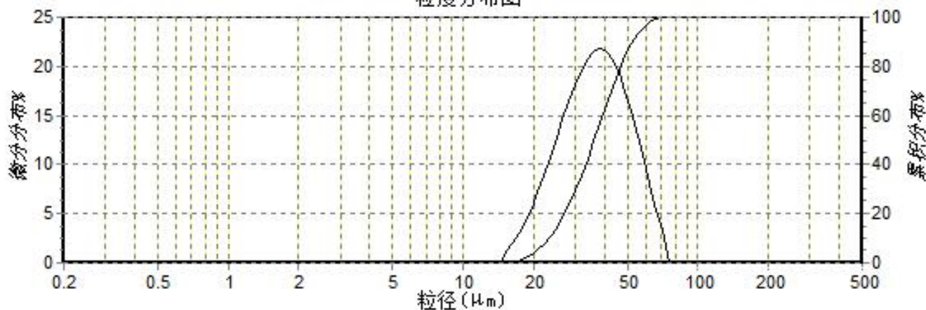
粒度分布图
