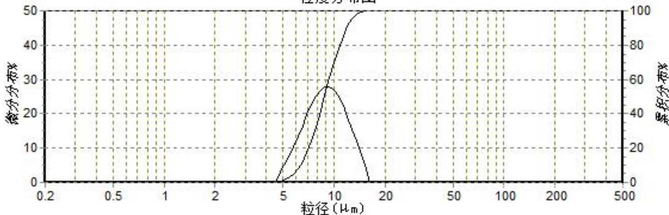
粒度分布图
